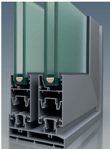
SISTEMA ELEVABLE CLÁSICA EXT45
