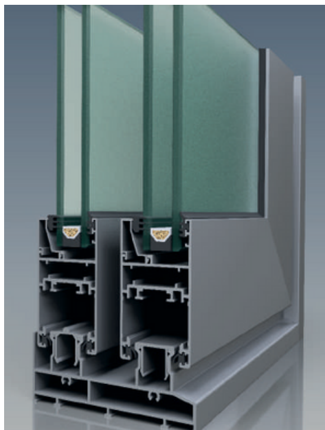
SISTEMA ELEVABLE LIVIANA EXT45
