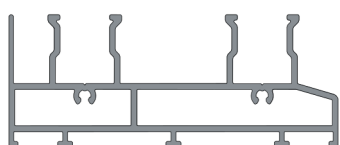
Contramarco Sup/Inf 2 vías
