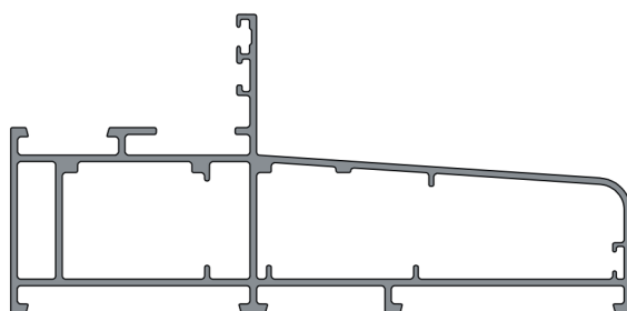
Contramarco Vidrio Fijo Corrediza Elevable
