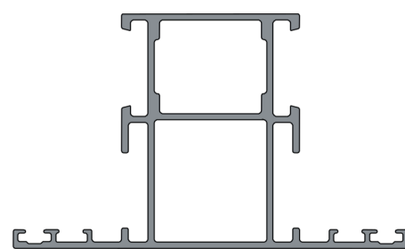
Marco División 45.00 mm
